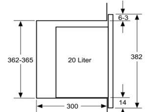
Maße in mm
